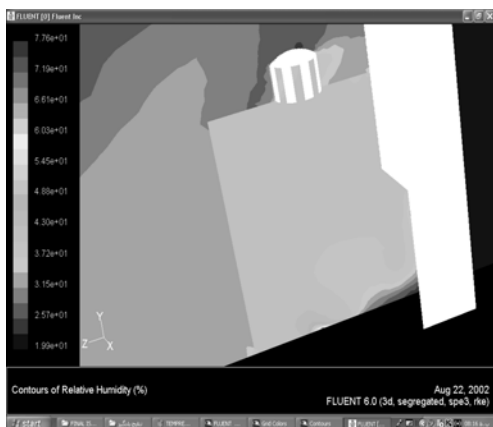
تصویر ۱۲- کانتور رطوبت نسبی در مقطع، مدل ۲
